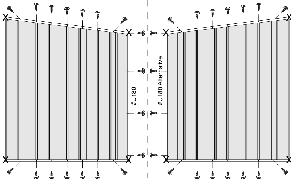
#U180 x 1 Left Door Frame
