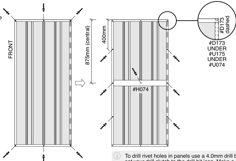
#H074 Door Bar
